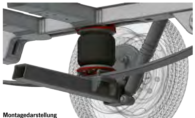
Montagedarstellung
